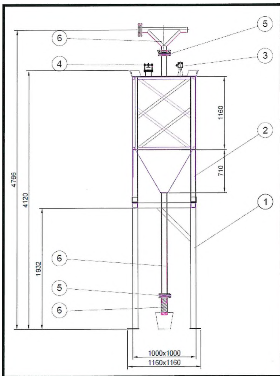
Obrázek 1.: náčrt koncového zásobníku písku.
