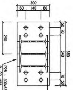
ČELNÍ DESKA MONTÁŽNÍHO STYKU 3 M 1:10
