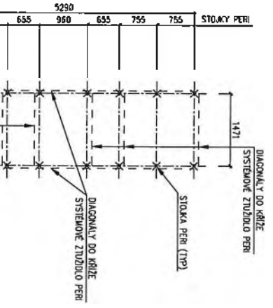
PŮDORYS STOLKŮ PERI M 1:50
