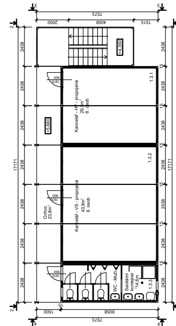
PŮDORYS 3.NP
