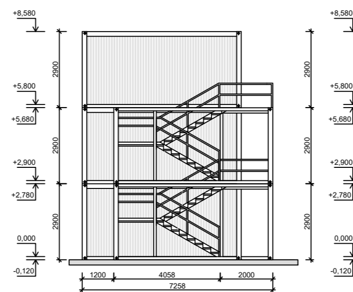
POHLED 3-3
