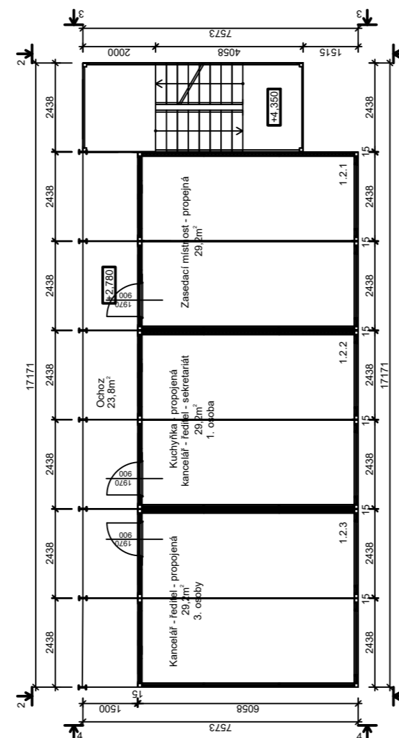
PŮDORYS 2.NP
