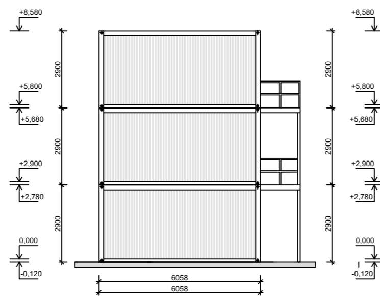
POHLED 4-4
