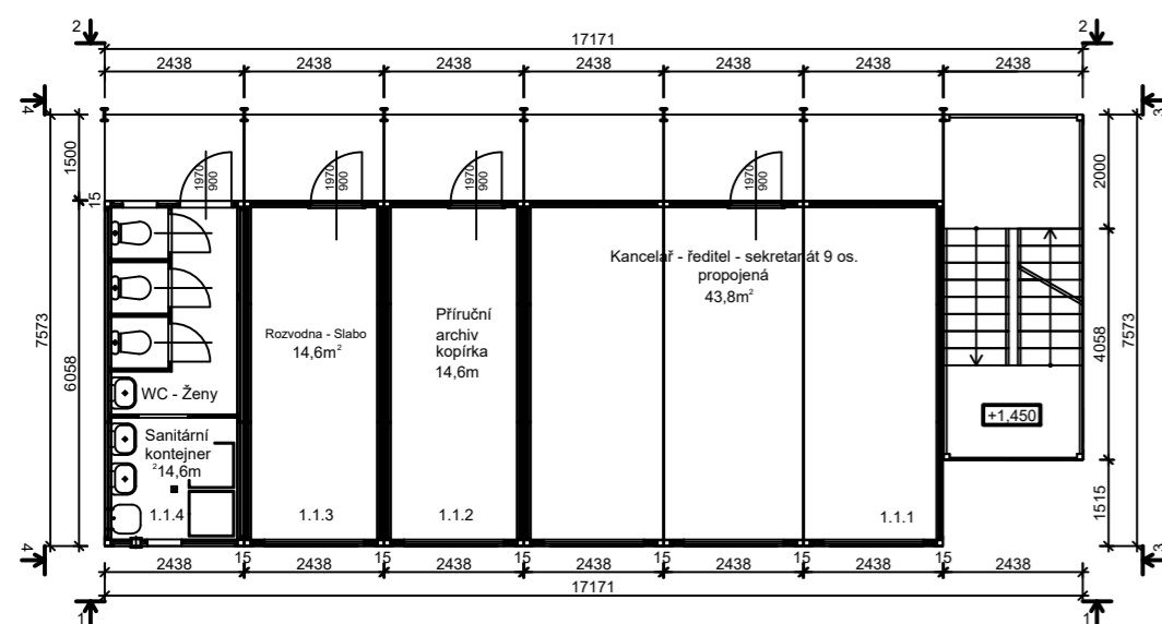
PŮDORYS 1.NP
