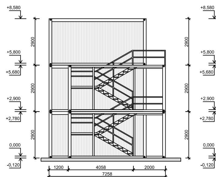
POHLED 3-3
