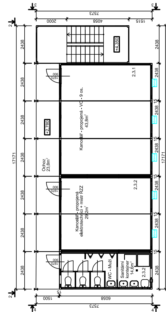
PŮDORYS 3.NP
