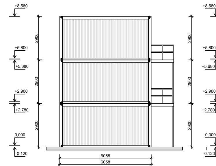
POHLED 4-4
