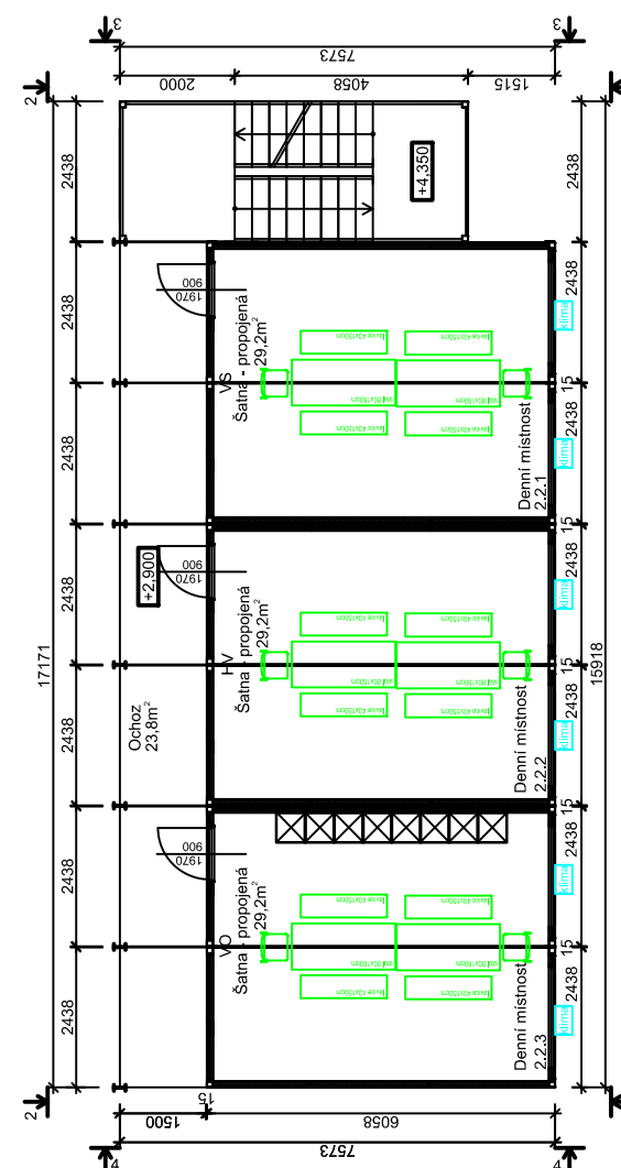
PŮDORYS 2.NP
